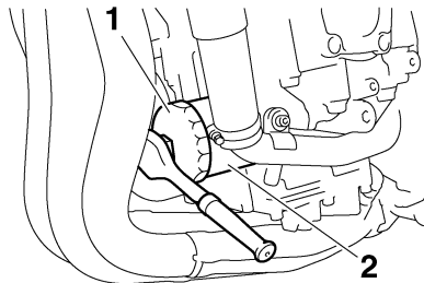
1. Llave del filtro de aceite 2. Cartucho del filtro de aceite
