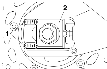
1. Marcas de alineación 2. Tensor de la cadena de transmisión
