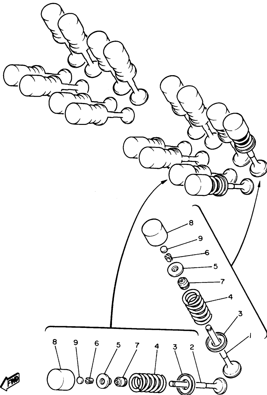
FIG. 4 VALVULA
